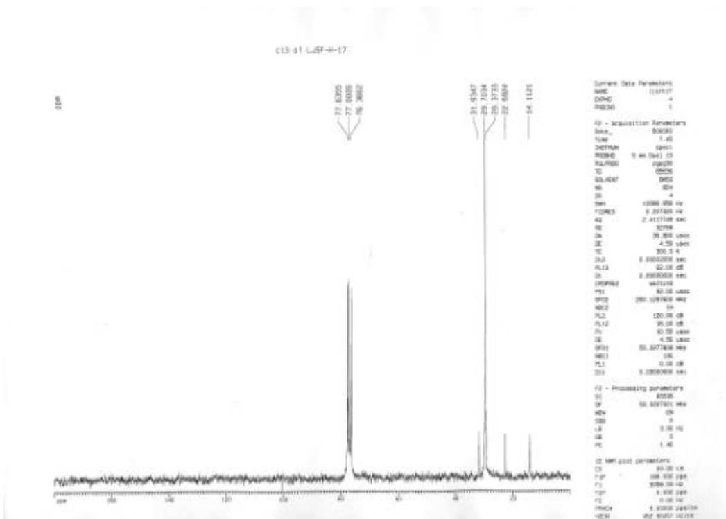
圖 5 : ^{13}\text{C} -NMR spectrum of compound II
